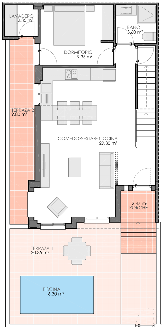
PLANTA BAJA
