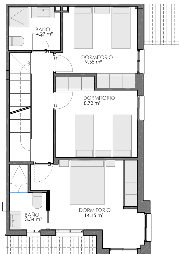
PLANTA PRIMERA
