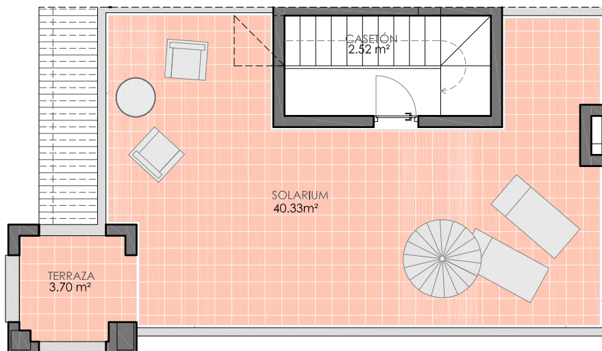
SOLARIUM
