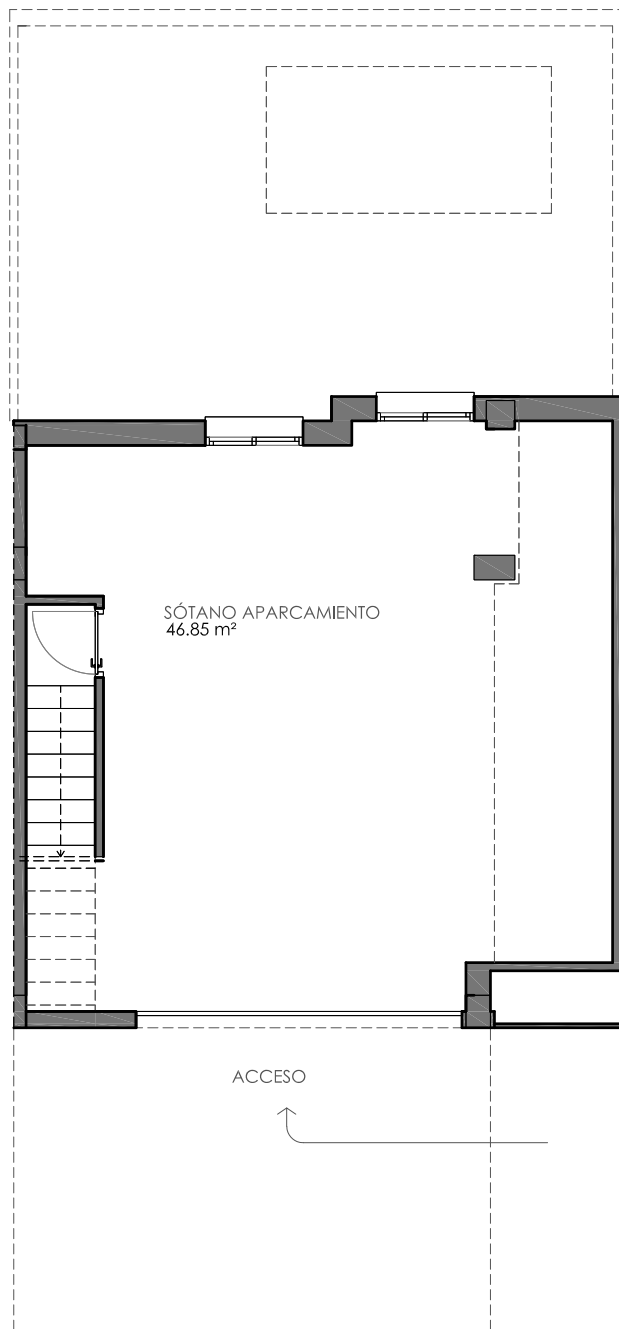
SÓTANO
