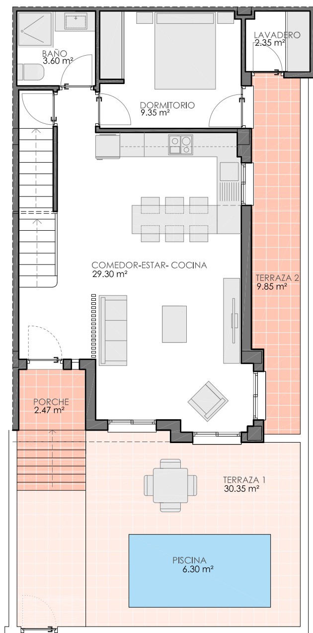
PLANTA BAJA
